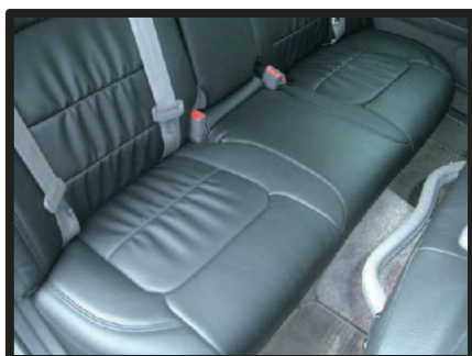
⑥座面は、背もたれ完成後に取り付けます。カバーの表面を整え、2列目座面の完成です。
