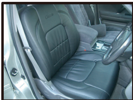
⑫サイドエアバッグ装備車は、サイドエアバッグの展開部分とシートカバーのSAB対応の縫い目部分が合っていることを確認して下さい。カバー表面を整え、運転席背もたれの完成です。助手席側も同様に取り付けます。
