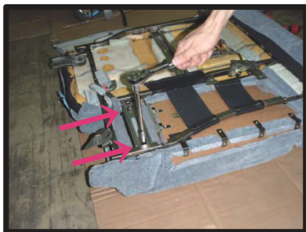
① 背もたれ裏側のアームレスト固定用ナットをラチェット等を使用して外します。
