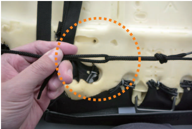
8 作った輪にもう片側のヒモを通して引きま す。
