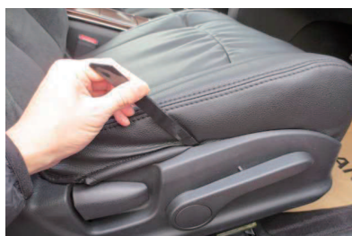
11 シート外側面のシートとプラスチック部の隙間に、ヘアなどを使用して生地を入れ込みます。
